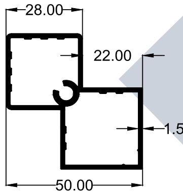
SECTION NO : 5068 WEIGHT : 0.924 (KG/M)
