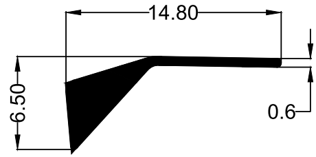
SECTION NO : 5054 WEIGHT : 0.059 (KG/M)
