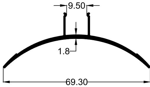
SECTION NO : 5046 WEIGHT : 0.380 (KG/M)
