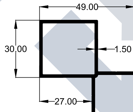
SECTION NO : 5282 WEIGHT : 0.616 (KG/M)
