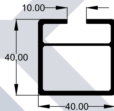
SECTION NO : 5254 WEIGHT : 0.939 (KG/M)
