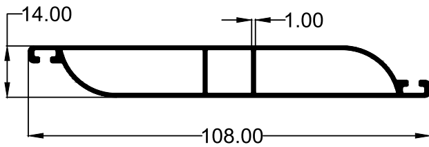
SECTION NO : 5062 WEIGHT : 0.707 (KG/M)
