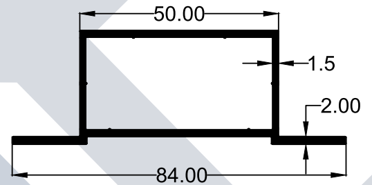
SECTION NO : 5025 WEIGHT : 0.870 (KG/M)
