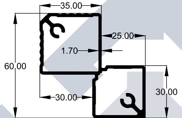
SECTION NO : 5124 WEIGHT : 1.23 (KG/M)
