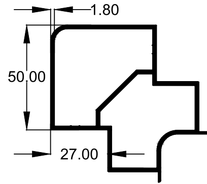
SECTION NO : 5122 WEIGHT : 1.52 (KG/M)
