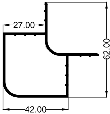
SECTION NO : 5028 WEIGHT : 0.755 (KG/M)
