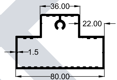
SECTION NO : 5069 WEIGHT : 1.25 (KG/M)
