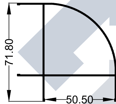
SECTION NO : 5143 WEIGHT : 0.718 (KG/M)
