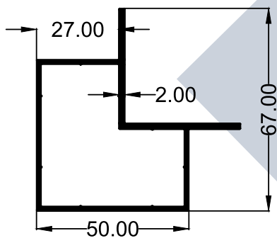
SECTION NO : 5024 WEIGHT : 1.03 (KG/M)
