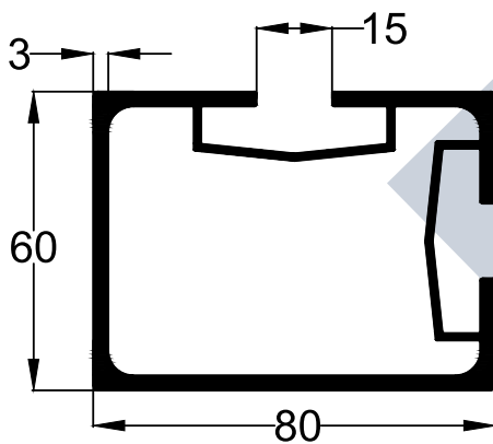
SECTION NO : 5130 WEIGHT : 2.43 (KG/M)
