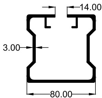
SECTION NO : 5057 WEIGHT : 2.69 (KG/M)
