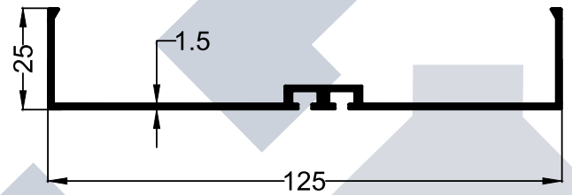
SECTION NO : 5066 WEIGHT : 0.819 (KG/M)
