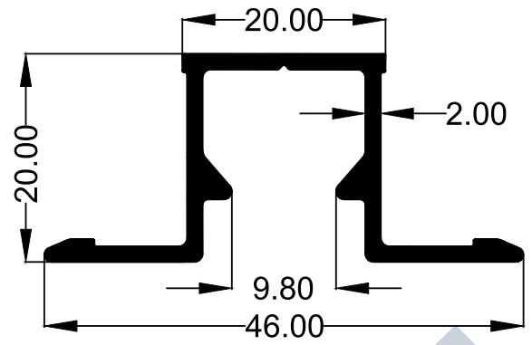
SECTION NO : 5146 WEIGHT : 0.393 (KG/M)
