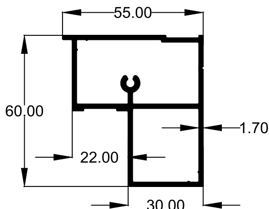
SECTION NO : 5127 WEIGHT : 1.26 (KG/M)
