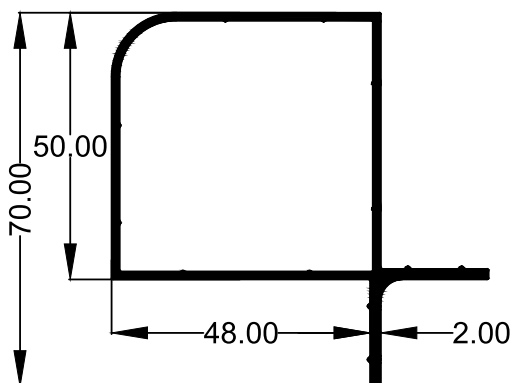
SECTION NO : 5085 WEIGHT : 1.000 (KG/M)
