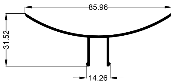
SECTION NO : 5149 WEIGHT : 0.403 (KG/M)
