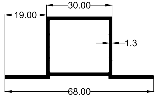
SECTION NO : 5021 WEIGHT : 0.550 (KG/M)
