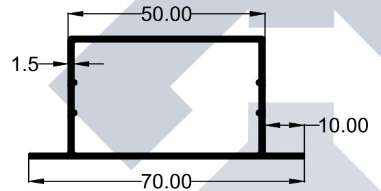
SECTION NO : 5065 WEIGHT : 0.727 (KG/M)
